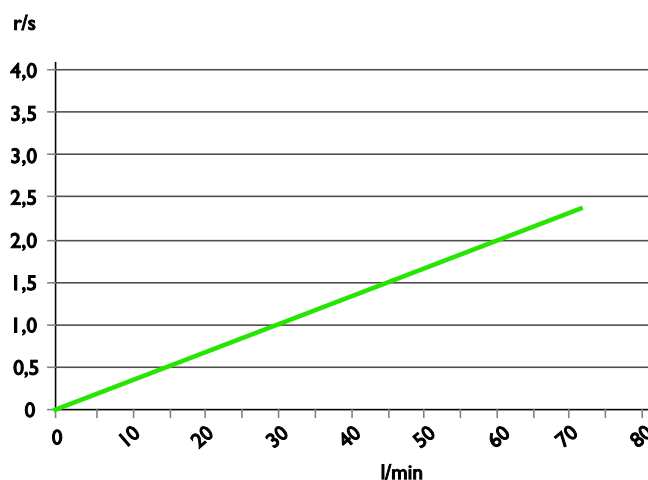
Graf 1 - Multifunktionsaggregatets rotationshastighet, varv per sekund
